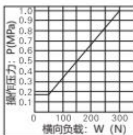
横向负载表
