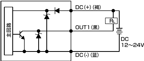
NPN输出
