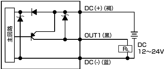
PNP输出
