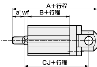
SSD(双作用·单活塞杆型)、SSD-T(耐热型)、SSD-F(微速型)、SSD-O(低速型)尺寸表
