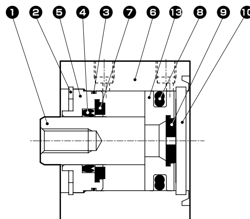
● SSD-16D~32D(双作用型)
