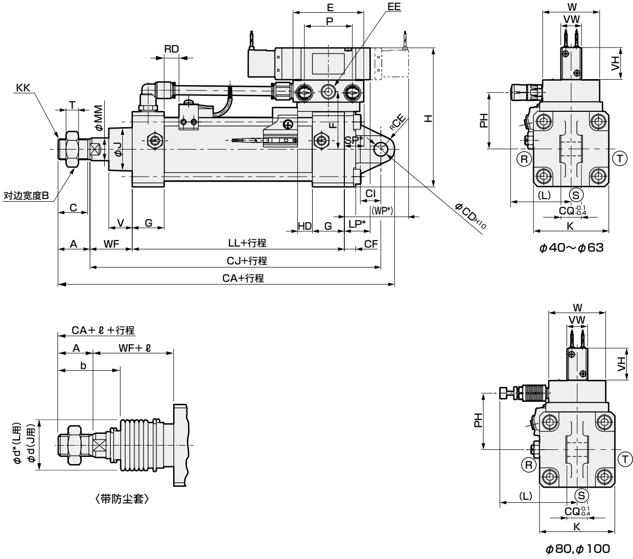
外形尺寸图
