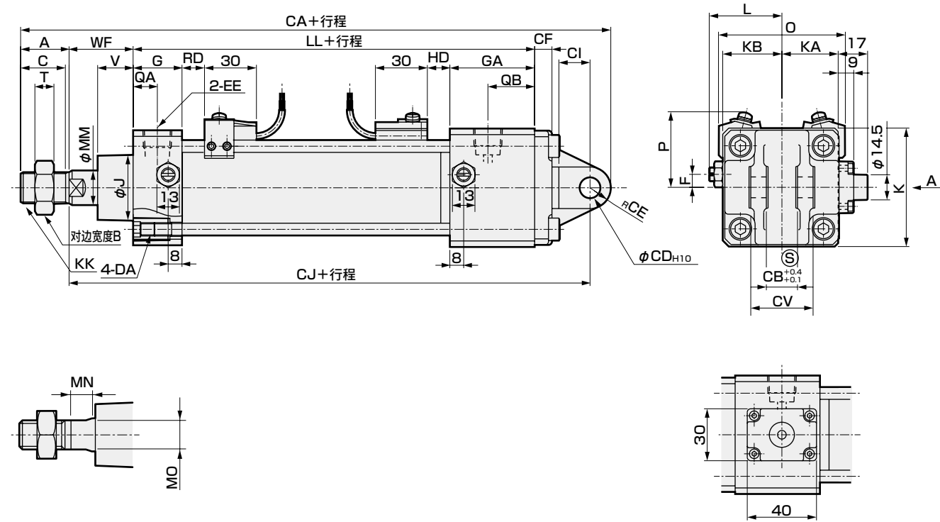
A向视图
