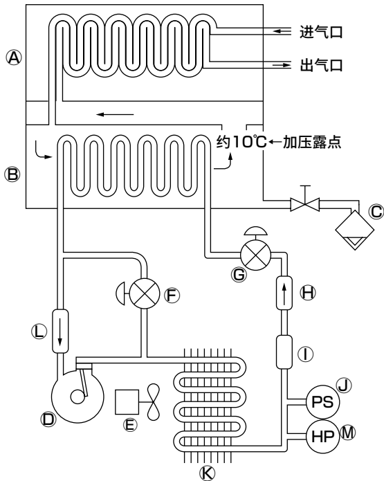
(系统图)
