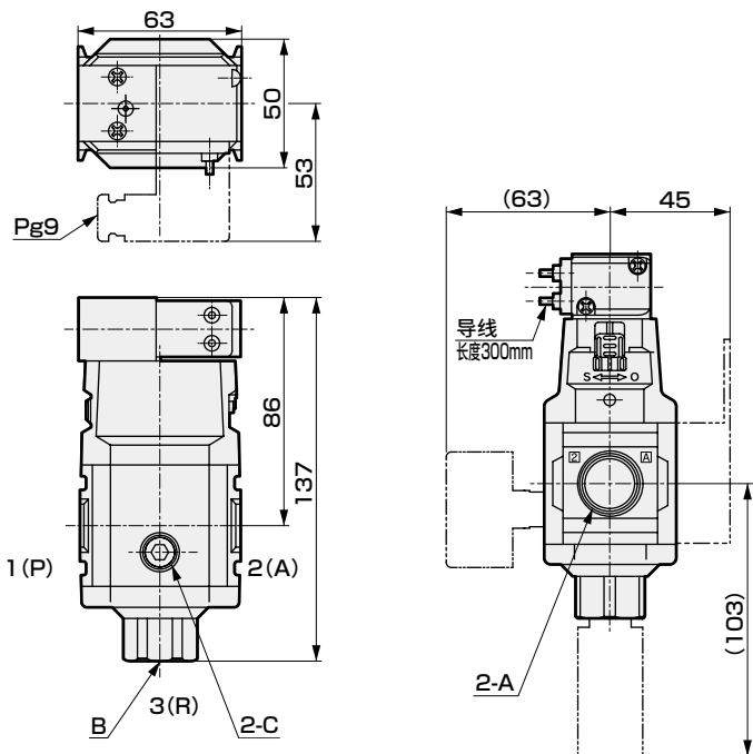
外形尺寸图
