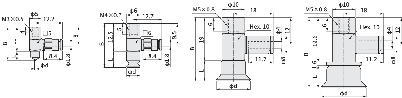
外形尺寸图(小型 固定式 抽真空口 横向 VSP-MB 快插接头型)
