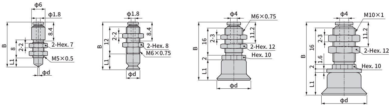
外形尺寸图(小型 固定式 抽真空口 向上 VSP-MA 快插接头型)
