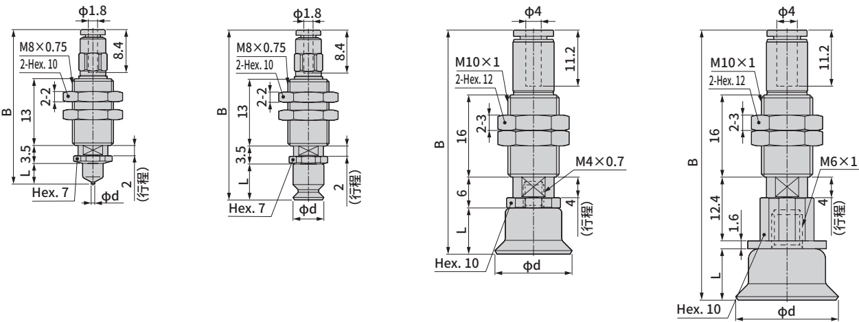
外形尺寸图(小型 缓冲式 抽真空口 向上 VSP-MC 快插接头型)
